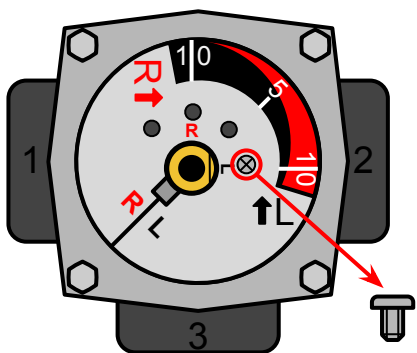
Position de la vis: repere L
