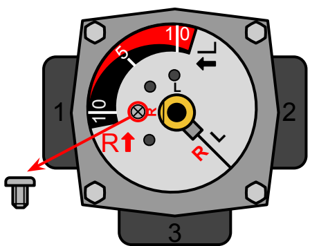
Position de la vis: repere R
