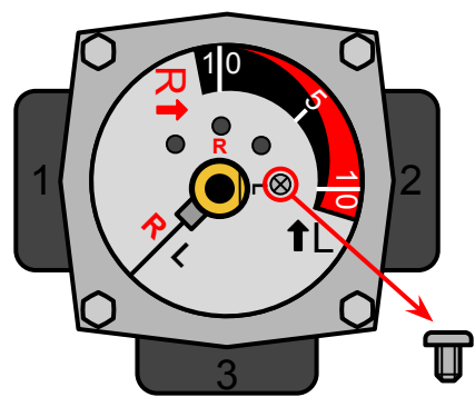
Position de la vis: repere L
