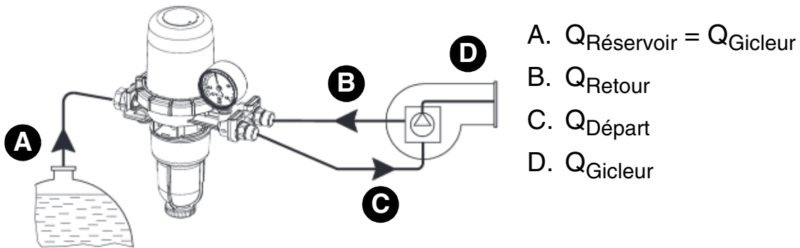
Figure 1: Fonctionnement FloCo-Top
