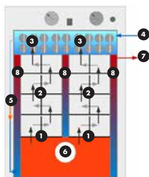
Schéma hydraulique chaudière et parcours des fumées - 24 kW
