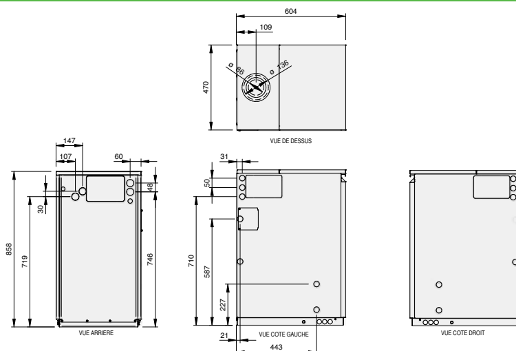
Dimensions chaudières Vortex Utility 18 kW et 24 kW
