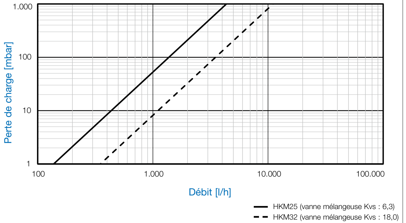
Courbe de perte de charge par rapport au débit FlowBox HKM25 et HKM32
